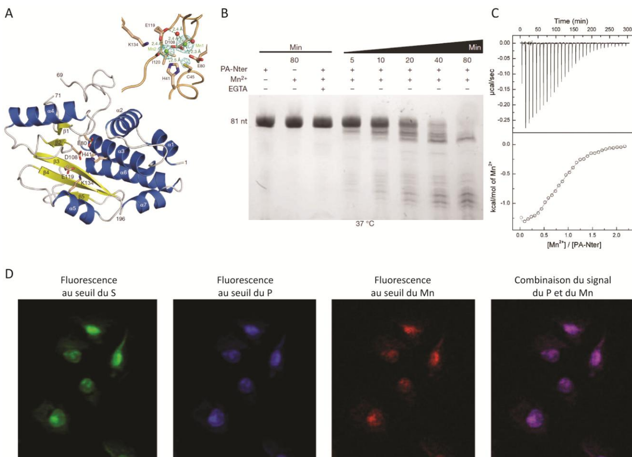
Figure 10: Caractérisation du domaine endonucléase isolé PA Nter . (A) Structure du domaine avec les hélices- \alpha représentées en bleu et les brins- \beta en jaune. L'encart supérieur montre la densité électronique des atomes de manganèse (sphères vertes) dans le site actif du domaine endonucléase. La carte de densité électronique fo-fc à partir de données de diffraction anormales collectées au seuil du manganèse est contournée à 3\sigma . (B) Activité nucléase de PA Nter . (C) Titration par microcalorimétrie de l'affinité de PA Nter pour le manganèse. (D) Cartographie du signal de fluorescence des rayons-X de différents éléments de cellules épithéliales alvéolaires humaines (A549). Figure adaptée de (Crépin et al. , 2010; Dias et al. , 2009a; Dias et al. , 2009b).
