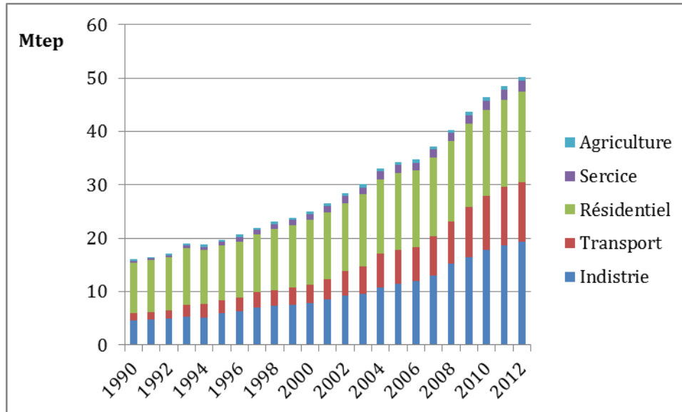
Graphique 1.5. Consommation de l'énergie finale par secteur de 1990-2012 9
