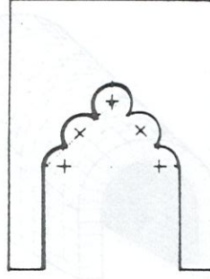
ARC POLYLOBÉ
