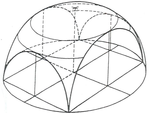
VOÛTE SPHÉRIQUE SUR PLAN BARLONG
