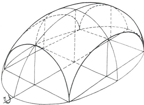
VOÛTE DOMICALE BARLONGUE (ELLIPSOÏDE)
