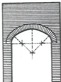
ARC EN ANSE DE PANIER - 3 CENTRES
