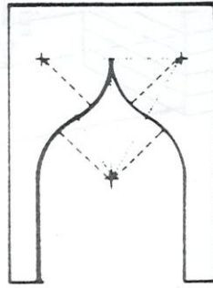
ARC FLAMBOYANT
