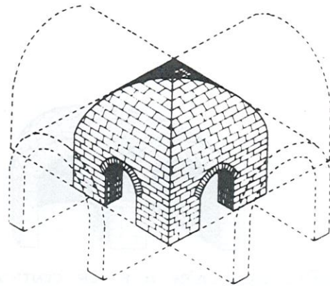
VOÛTE EN ARC DE CLOÎTRE
