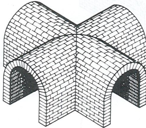
INTERSECTION DE DEUX BERCEAUX DE MÊME MONTÉE
