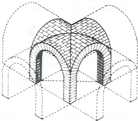
VOÛTE D'ARÊTE
