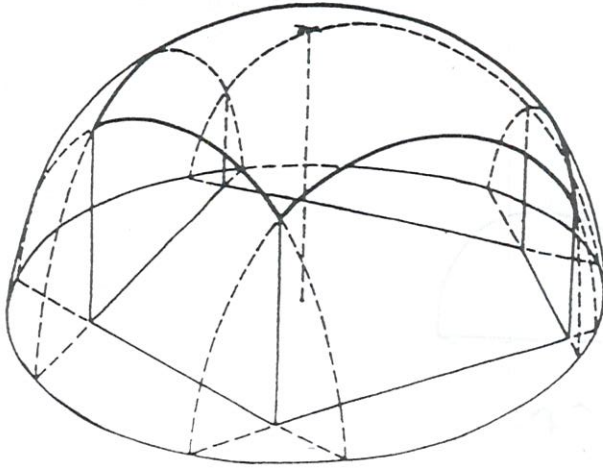
VOÛTE SPHÉRIQUE SUR PLAN POLYGONAL QUELCONQUE
