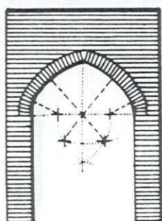
ARC TUDOR ESPAGNOL 4 CENTRES
