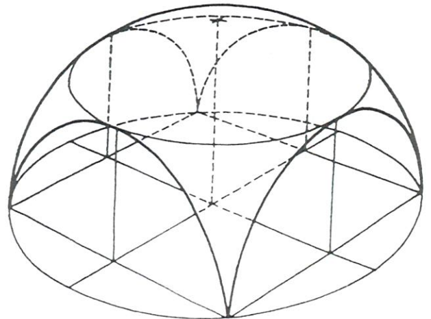
VOÛTE SPHÉRIQUE À PENDENTIFS
