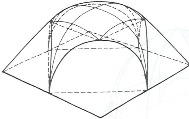
VÔTE EN TROMPES D'ANGLE
