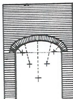
ARC EN ANSE DE PANIER - 5 CENTRES
