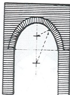
ARC EN ELLIPSE HAUTE - 2 Foyers
