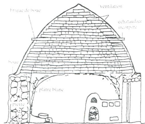
Coupe d'une maison à coupole.
