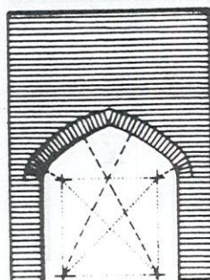
ARC TUDOR ESPAGNOL AIGU : 4 CENTRES
