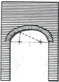
ARC EN ELLIPSE BASSE - 2 Foyers
