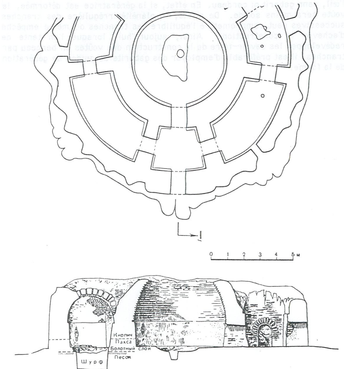
Рис. 101. Купольный мавзолей Баланды 2. План и разрез.
