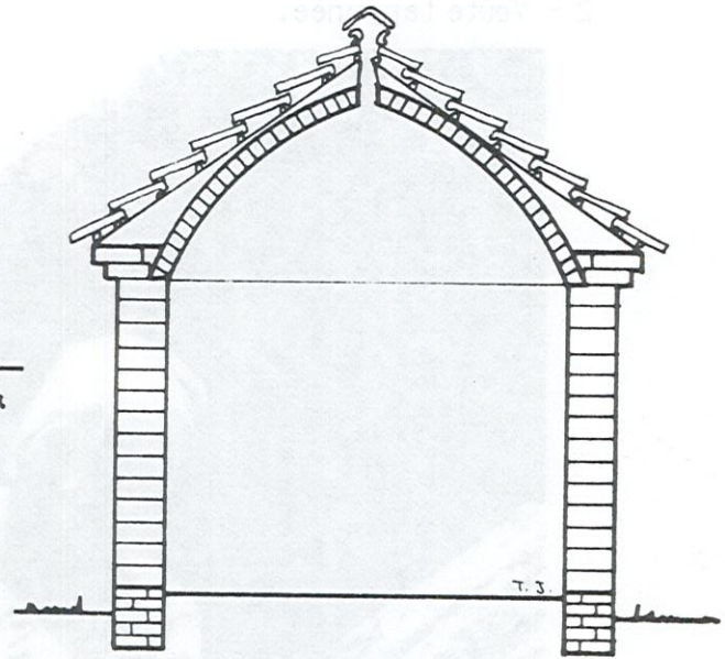
_COUPE A'A_
