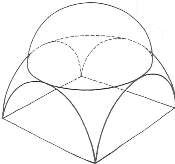
COUPOLE HÉMISPHERIQUE SUR PENDENTIFS
