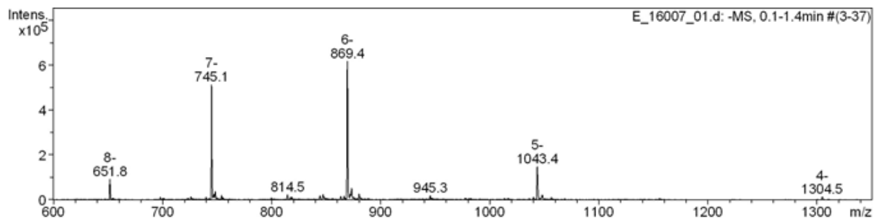
Fig. S16. ESI mass spectrum of oligonucleotide 7
