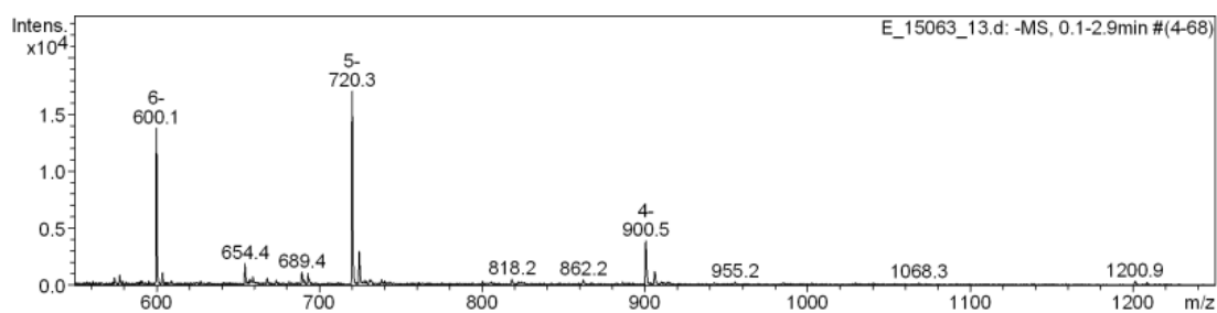
Fig. S12. ESI mass spectrum of oligonucleotide 6
