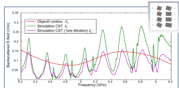
Figure 9. Comparaison entre l'objectif et les résultats obtenus sans itération et après une itération.
