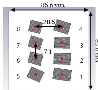
Figure 8. Tag sans puce simulé avec CST Microwave Studio 2014 (solver temporel).
