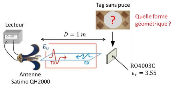
Figure 3. Configuration de mesure donnée à l'avance pour le problème de synthèse.
