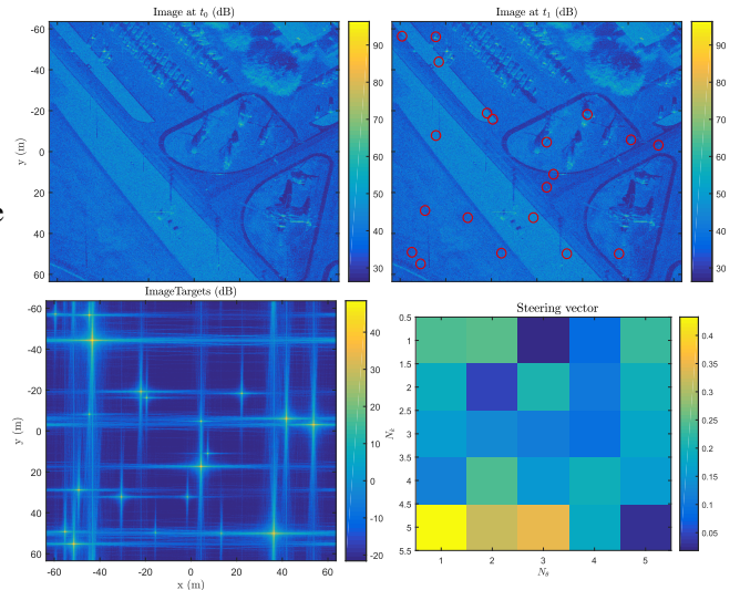
FIGURE 3 – Exemple de changement (RSB : entre [0; 30] dB, position : aléatoire). Haut-gauche : Image I. Haut-droit : Image J. Bas-gauche : Image des cibles. Bas-droit : Signature d'une cible.
