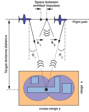
FIGURE 1 – Géométrie d'acquisition. Un réflecteur est vu selon deux angles d'illuminations
