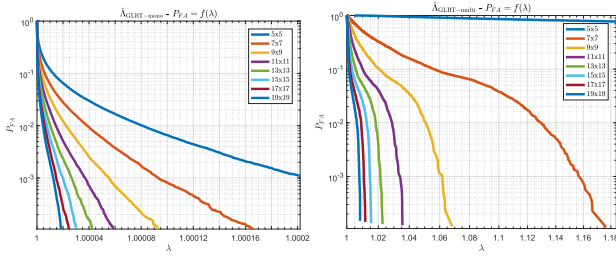
FIGURE 4 – P_{FA} = f(\lambda) (calculé sur 1500 \times 1500 échantillons). Gauche : \hat{\Lambda}_{GLRT-mono} . Droite : \hat{\Lambda}_{GLRT-multi} .
