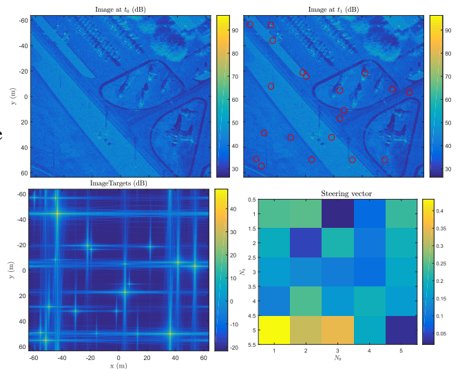
FIGURE 3 – Exemple de changement (RSB : entre [0; 30] dB, position : aléatoire). Haut-gauche : Image I. Haut-droit : Image J. Bas-gauche : Image des cibles. Bas-droit : Signature d'une cible.
