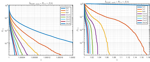
FIGURE 4 – P_{FA} = f(\lambda) (calculé sur 1500 \times 1500 échantillons). Gauche : \hat{\Lambda}_{GLRT-mono} . Droite : \hat{\Lambda}_{GLRT-multi} .
