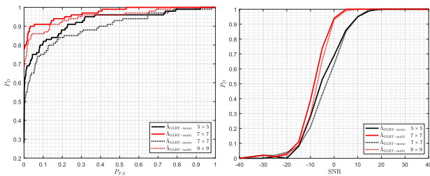
FIGURE 6 – Gauche : P_D = f(P_{FA}) (100 réalisations, SNR = -5dB, position aléatoire). Droite : P_D = f(SNR) (100 réalisations, P_{FA} = 10^{-3} , position aléatoire).
