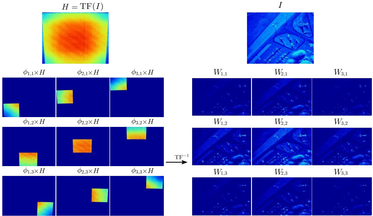
FIGURE 2 – Exemple de décomposition avec N_k, N_\theta = 3, 3
