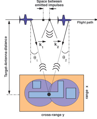
FIGURE 1 – Géométrie d'acquisition. Un réflecteur est vu selon deux angles d'illuminations
