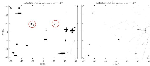
FIGURE 5 – Détection à P_{FA} = 10^{-3} . Gauche : \hat{\Lambda}_{GLRT-multi} ( 7 \times 7 ). Droite : \hat{\Lambda}_{GLRT-mono} ( 5 \times 5 ).
