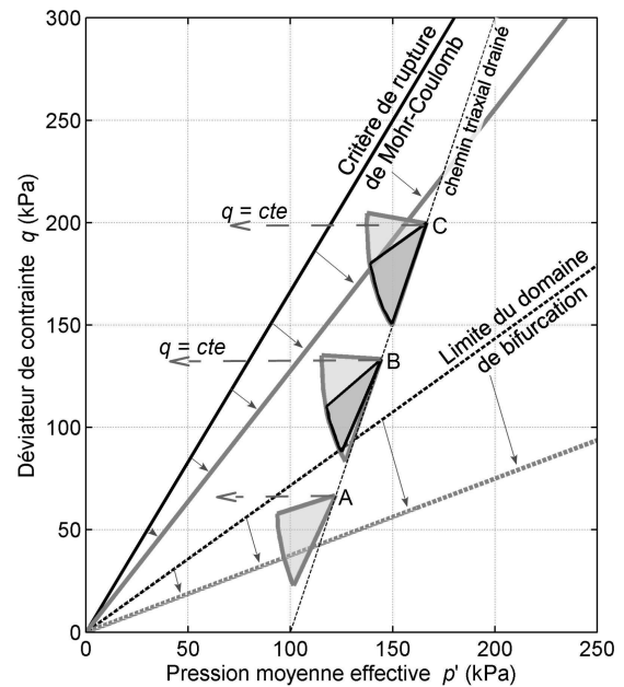
FIGURE 8: CHANGEMENT DU CRITÈRE DE MOHR-COULOMB, DE LA LIMITE INFÉRIEURE DU DOMAINE DE BIFURCATION, ET DES CÔNES DE DIRECTIONS INSTABLES POUR UNE TRANSITION D'UN SABLE D'HOSTUN D'UN ÉTAT DENSE (TRACÉS NOIRS) VERS UN ÉTAT LÂCHE (TRACÉS GRIS ÉPAIS), D'APRÈS [14]
