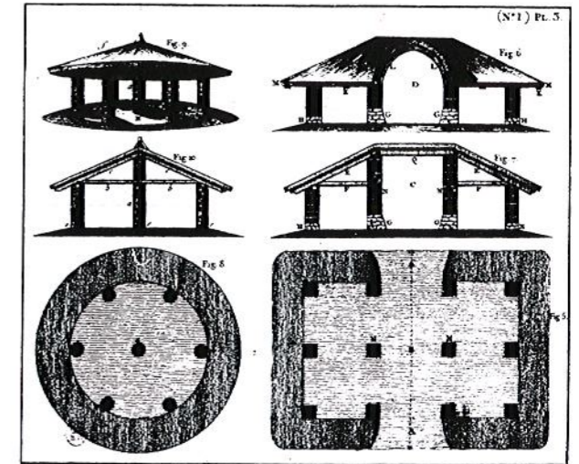
Fig. 12 : Modèle de séchoir en forme de halle avec piliers en pisé. In "Les erreurs de mon siècle sur l'agriculture", 1794.
