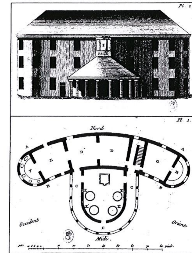
Fig. 13 : Modèle de chais et vendangeoir en pisé avec maison de vigneron. In "Le joyeux vigneron à ses vendanges", 1810.
