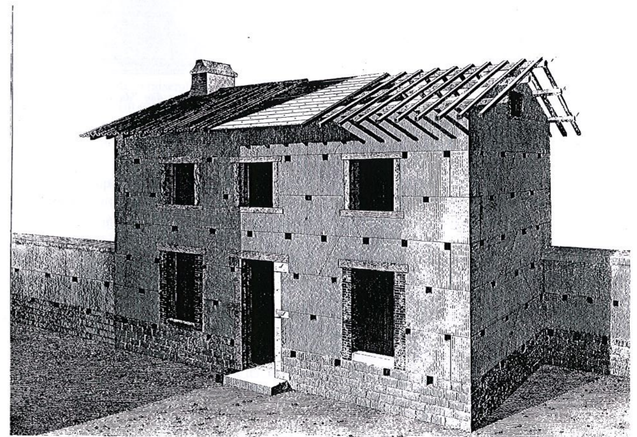
Fig. 3 : Modèle de maison économique en pisé. In "Traité de l'Art de Bâtir" de Jean-Baptiste Rondelet, édition de 1840.
